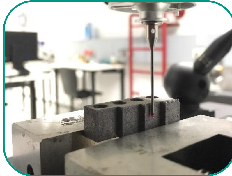
Taktile Koordinatenmesstechnik
